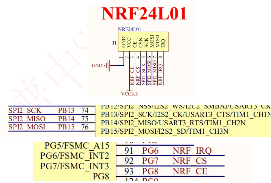
图 1.2.1 NRF24L01 模块接口与开发板连接原理图
